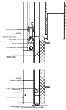
06 DOOR HEAD - SILL TYP SCALE: 1-1/2" = 1'
