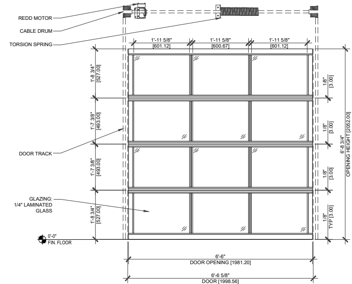
06 ELEVATION SCALE: 3/4" = 1'
