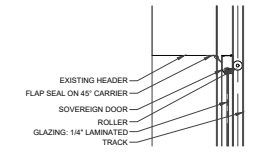
07 HEAD TYP SCALE: 1-1/2" = 1'
