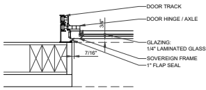
03 JAMB DETAIL SCALE: 1-1/2" = 1'
