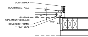
04 JAMB DETAIL SCALE: 1-1/2" = 1'
