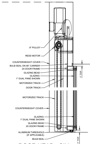
06 DOOR HEAD - SILL SCALE: 1-1/2" = 1'
